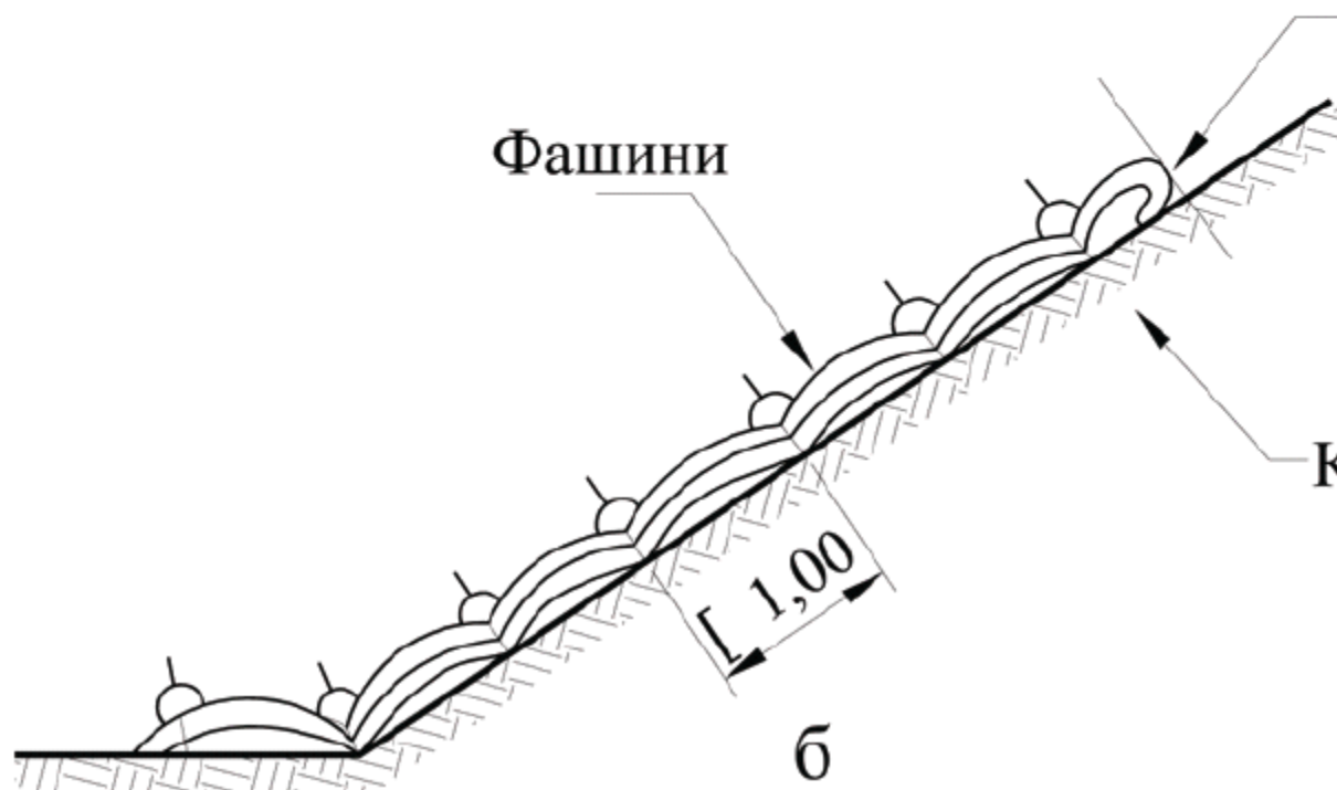
Фиг. 2. Укрепване на откоси с фашины
