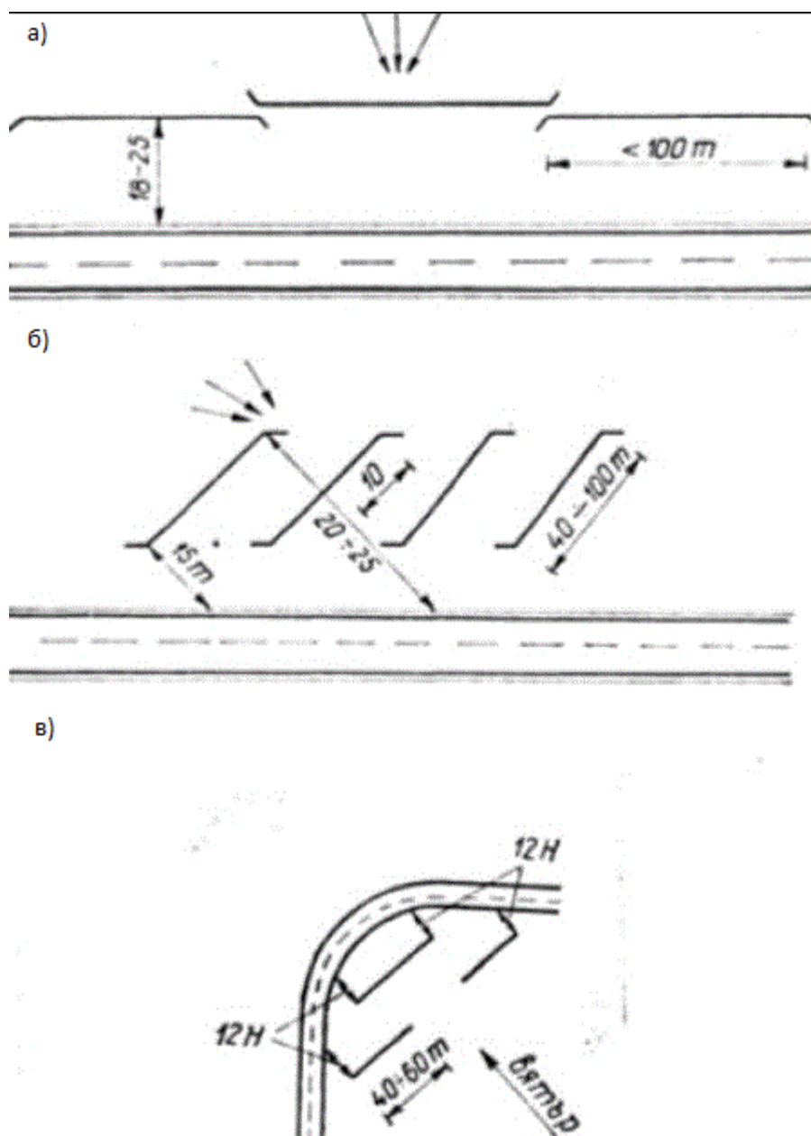
Фиг. 4. Разполагане на снегозащитни огради в зависимост от посоката на вятъра: а) успоредно на пътя; б) косо на пътя; в) в крива
