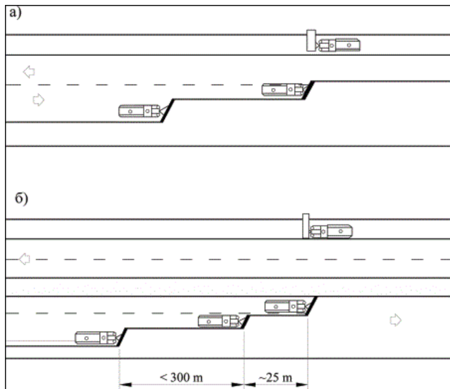
Фиг. 6. Схеми на патрулно снегопочистване:
